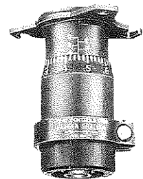
アジャスター (目盛0.02、0.1、1%、調整範囲±0.25%)
